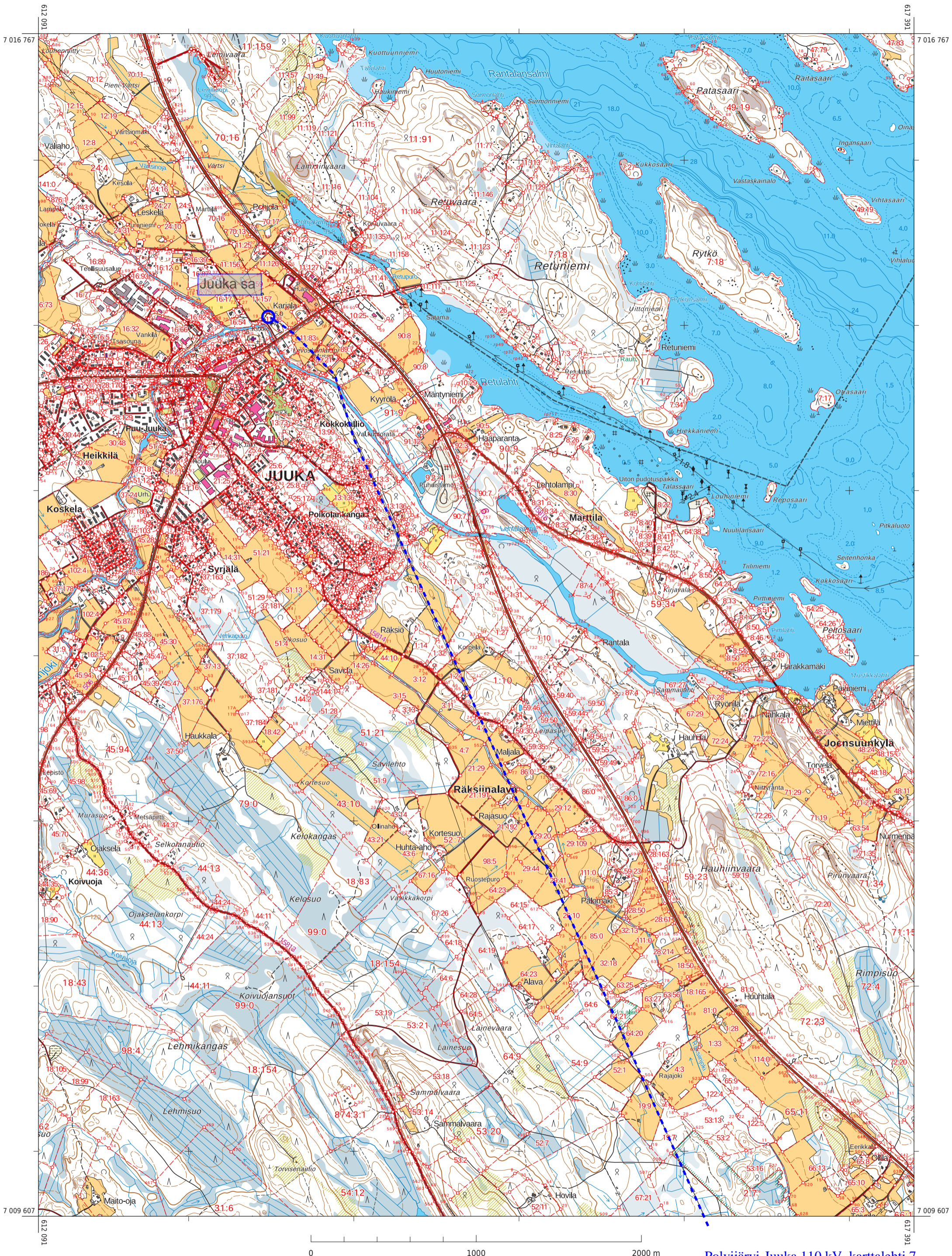
Polvijärvi-Juuka 110 kV, karttalehti 7
